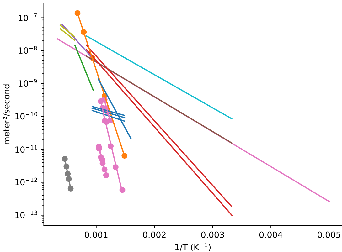
Tungsten diffusivity
